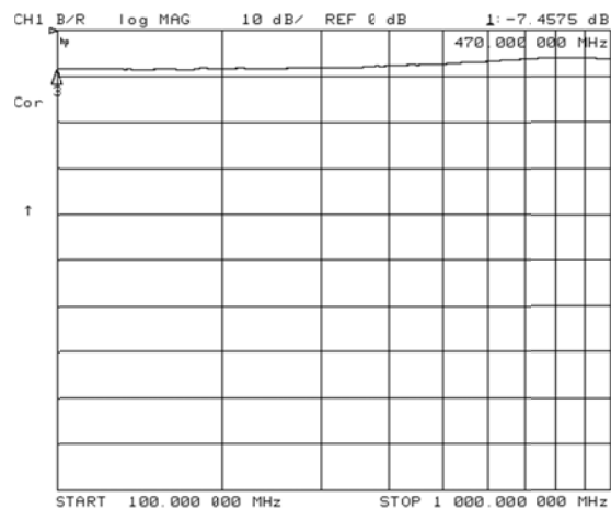
Grunddämpfung: Anschlüsse A–D zu X
