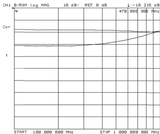
Entkopplung: Anschlüsse A/B und C/D (Marker 1+2), A/D und B/C (Marker 3+4)
